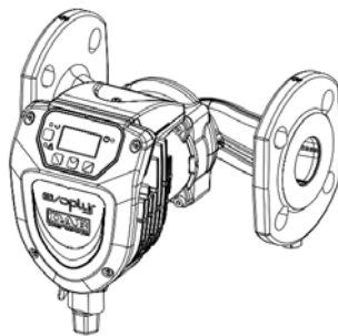
Abbildung 2: Installation an horizontalen Leitungen
