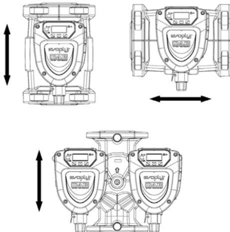
Afbeelding 1: montagepositie
