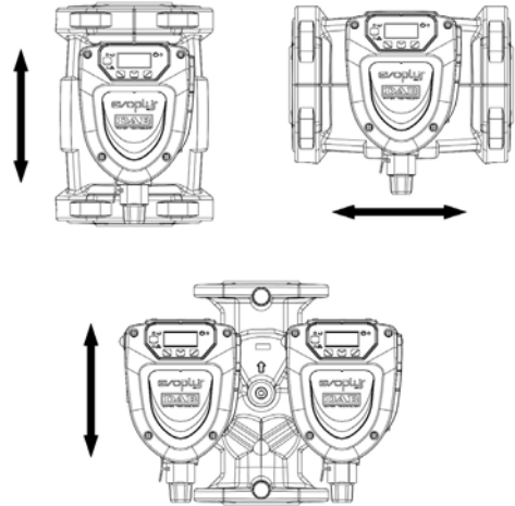
Resim 1: Montaj pozisyonu
