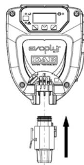
Figura 4: Connessione connettore di alimentazione
