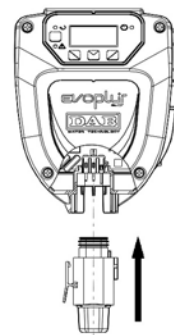
Rys. 4: Połączenie łącznika zasilania
