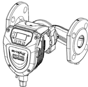
Figura 2: Instalación en tuberías horizontales
