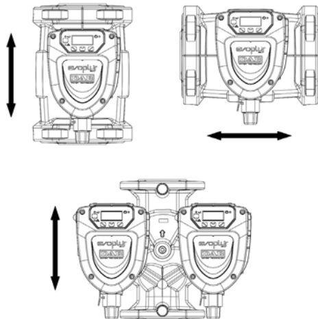
Obr. 1: Poloha montáže
