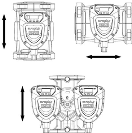
Rys. 1: Pozycja montażu
