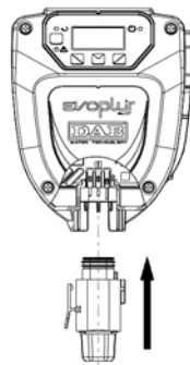
Figura 4: Conexión del conector de alimentación
