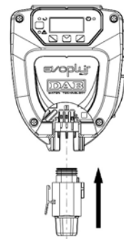
Figura 4: Conexiune conector de alimentare
