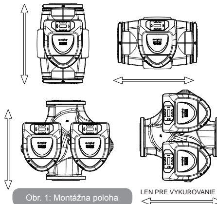
Obr. 1: Montážna poloha
