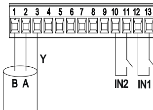
Slika 7: Snemljiva 13-polna priključna sponka: digitalni vhodi in MODBUS
