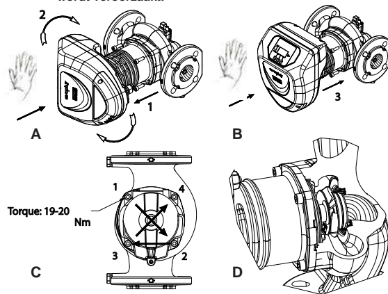
Afbeelding 2: Montage-instructies motorblokken
