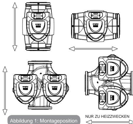
Abbildung 1: Montageposition
