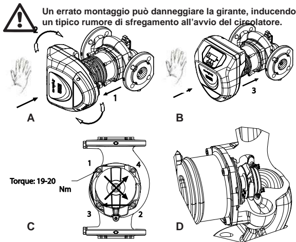
Figura 2: Istruzione di montaggio teste motore
