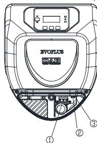
Kuv. 4: Sähköliitännät (etu)
