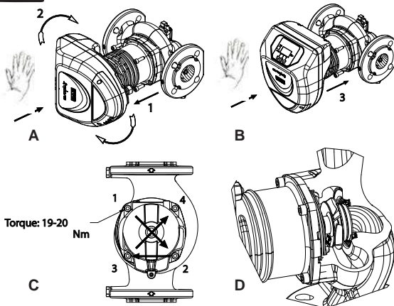
Figura 2: Instruções de montagem cabeças motor
