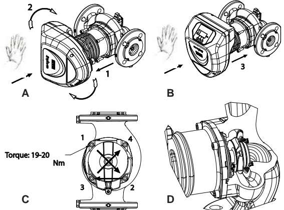
Resim 2: Motor kafaları montaj talimatları
