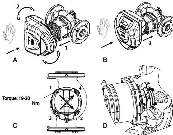
2 pav. Variklio galvučių įrengimo instrukcija
