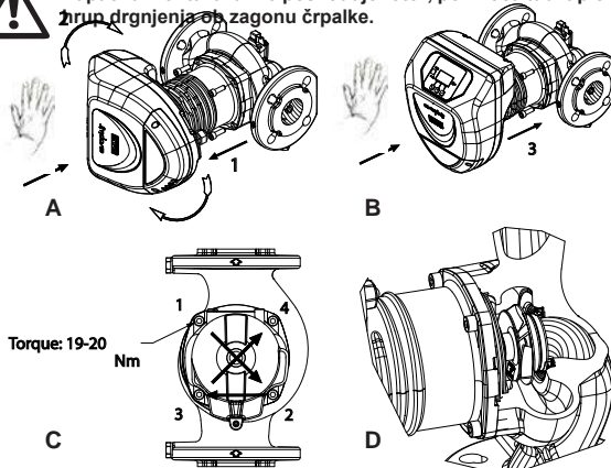
Slika 2: Navodilo za montažo glave motorja
